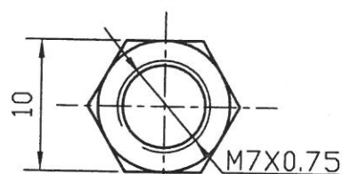
NUT 1PC
